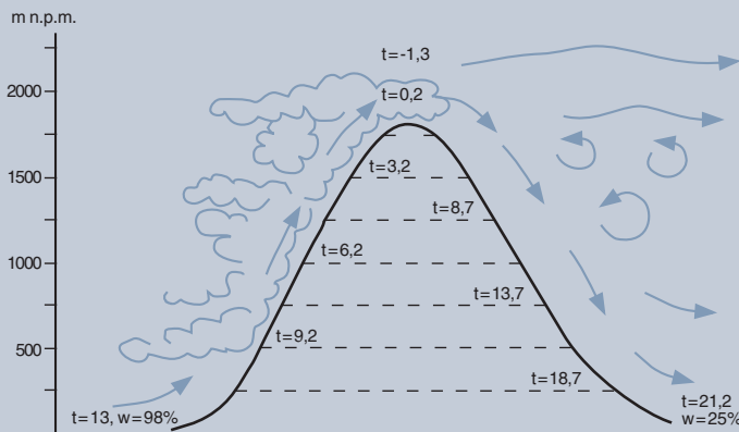
1. Schemat zjawisk zachodzących w czasie trwania wiatru halnego (rys. Igor J. Zaleski)
